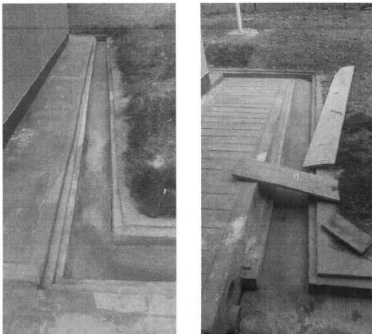
Foto 01: Tambo Cochatucoj con drenaje de evacuación de agua expuesto, sin rejas de protección.
